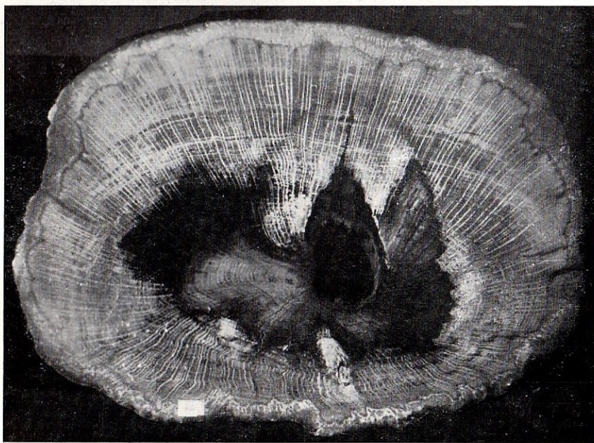
Sezione di tronco di legno silicizzato (diametri 23 e 31 cm.) di Holbrook, Arizona: si noti la perfetta conservazione degli anelli e soprattutto dei raggi midollari. La tessitura del legno è conservata in pieno, ma la sostanza organica è stata sostituita particella per particella da silice apportata da acque. Il campione è conservato nel Museo dell'Istituto di Mineralogia e Petrografia dell'Università di Bologna.
