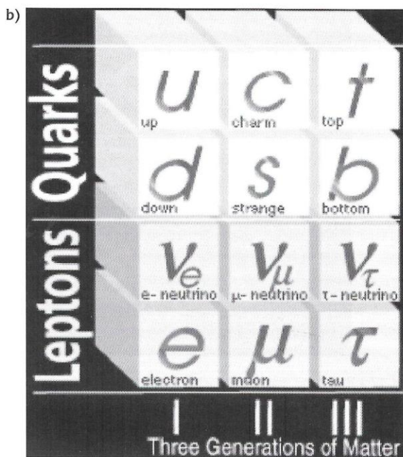
Fig. 15 – (a) I costituenti della materia, vuoto dovunque? (b) I costituenti ultimi.
