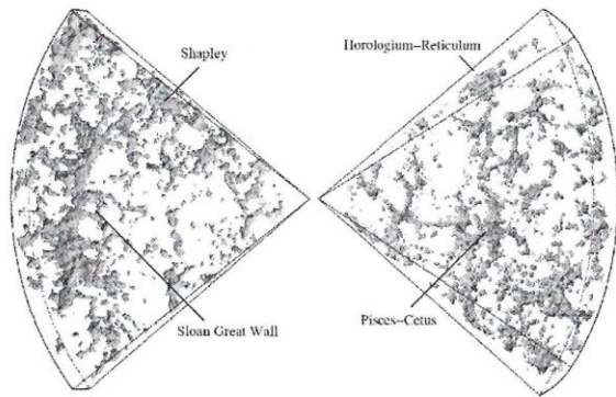
Fig. 4 – Struttura dell'universo a grande scala. Ogni puntino è una galassia (dal catalogo Sloan).
