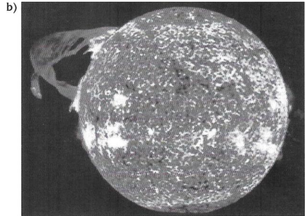
Fig. 2 – (a) Il telescopio ottico Hubble in orbita attorno alla terra. (b) Il sole: notare le protuberanze.
