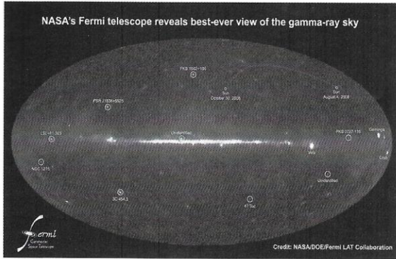
Fig. 12 – Il centro della nostra galassia osservato in raggi gamma.
