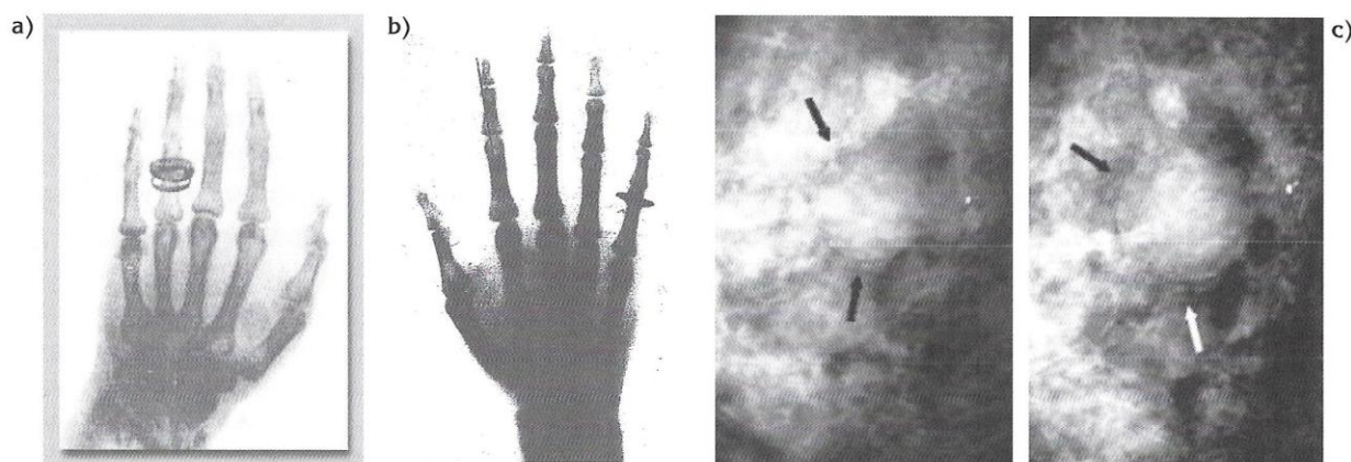
Fig. 16 – (a,b) Radiografie di una mano. (c,d) Mammografie a raggi X convenzionale (a sinistra) e con luce di sincrotrone (a destra). Le frecce indicano un'opacità rotondeggiante e ben riconoscibile a destra, dove è visibile un contorno netto che orienta verso la benignità del nodulo osservato.
