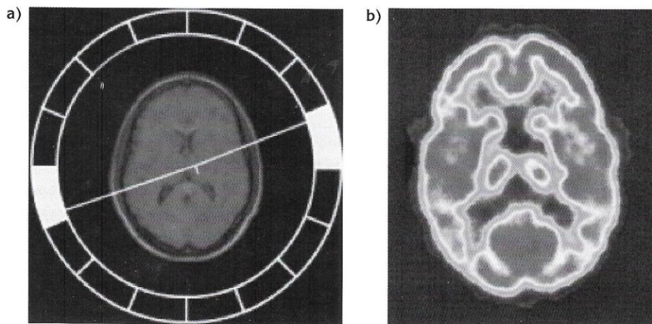
Fig. 18 – (a) Rappresentazione del funzionamento della PET [10]. (b) Tipica scansione PET di un cervello sano.
