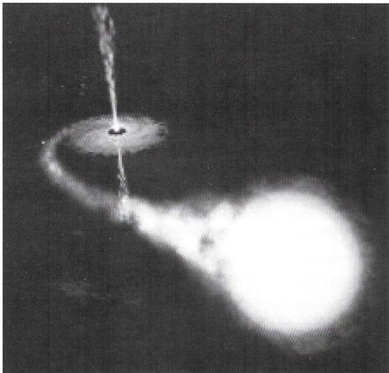
Fig. 10 – Schema illustrativo del microquasar GRO J 1640-40.
