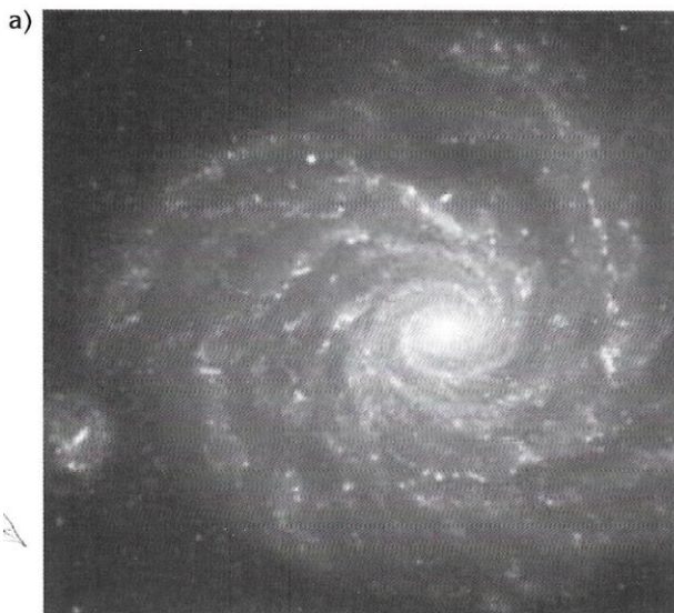
Fig. 3 – (a) La galassia spirale NGC 1232 fotografata da VLT Antu, ESO. (b) I telescopi ottici dell'ESO in Cile; i 4 telescopi usati insieme hanno un potere risolutivo pari a quello di un telescopio con le dimensioni qui viste in scuro. I 3 "piccoli telescopi" in basso ai vertici di un triangolo, se usati insieme sono equivalenti ad un telescopio delle dimensioni della circonferenza tratteggiata in bianco.
