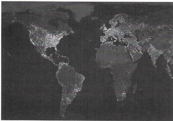
Fig. 13 – La luce emessa di notte dalle nostre città [11].
