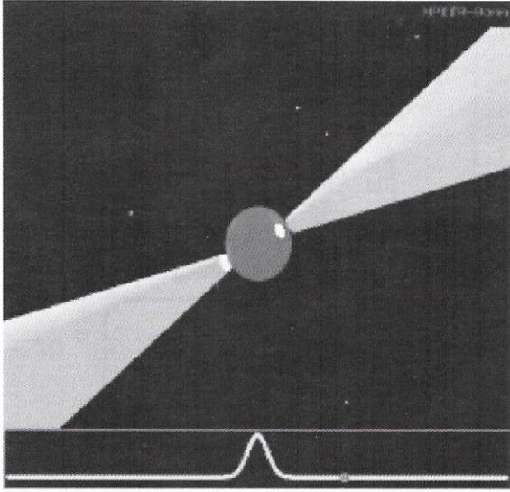
Fig. 8 – Schema del "Radiofaro" di una stella
