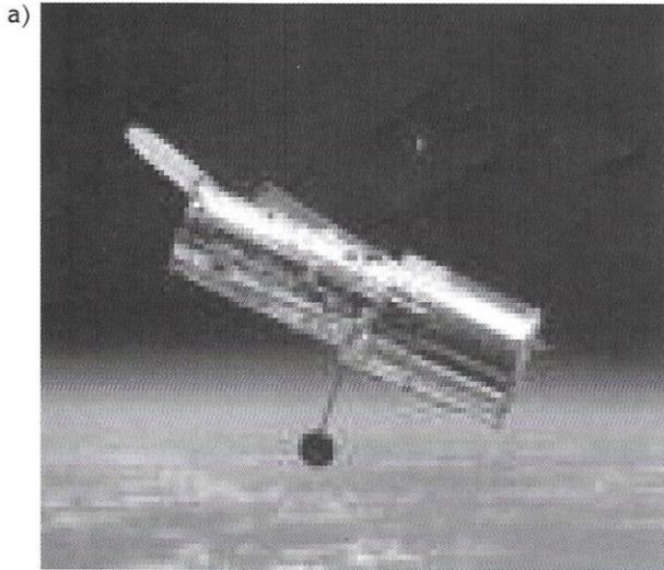
Fig. 2 – (a) Il telescopio ottico Hubble in orbita attorno alla terra. (b) Il sole: notare le protuberanze.
