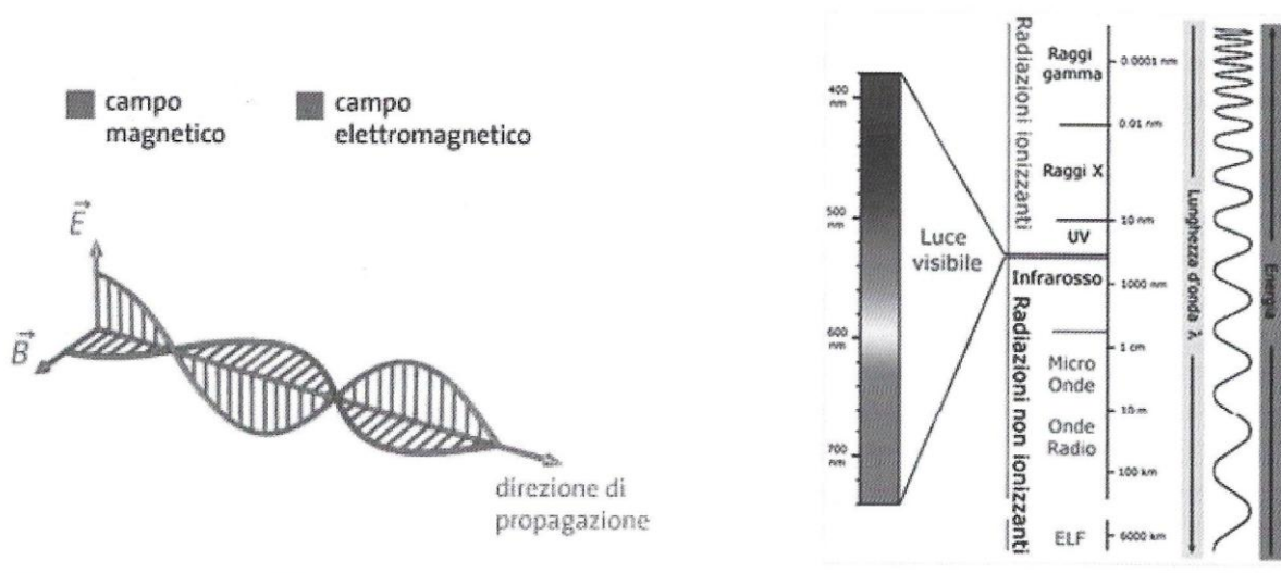
Fig. 5 – (a) Prospettiva della propagazione di un'onda elettromagnetica (O. E.). (b) Lo spettro delle onde E.M.
